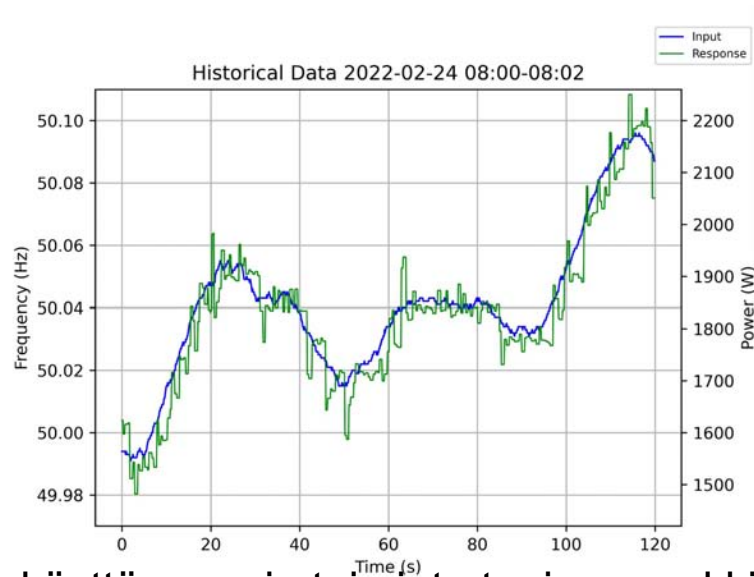
Kuva 1: käyttöreservin toiminta taajuusmarkkinoilla 24.2.2022
